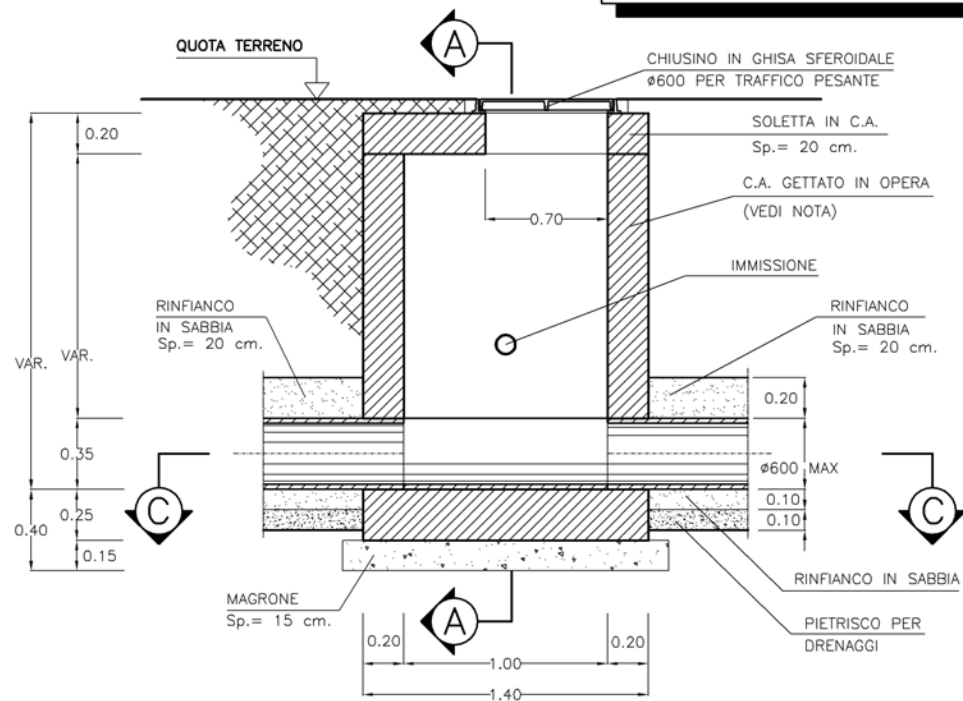
SEZIONE B-B 1:25
