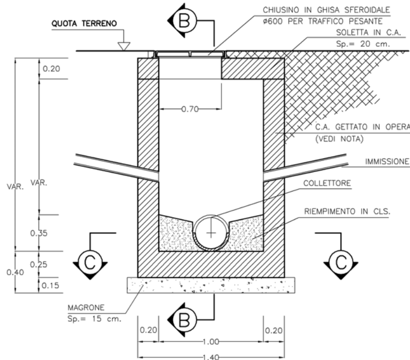
SEZIONE A-A 1:25
