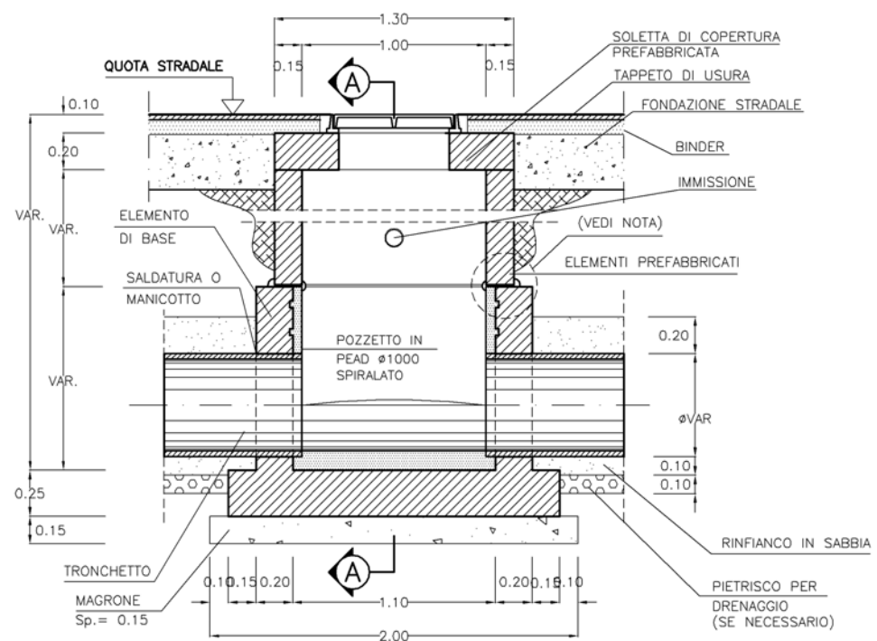
SEZIONE B-B 1:25
