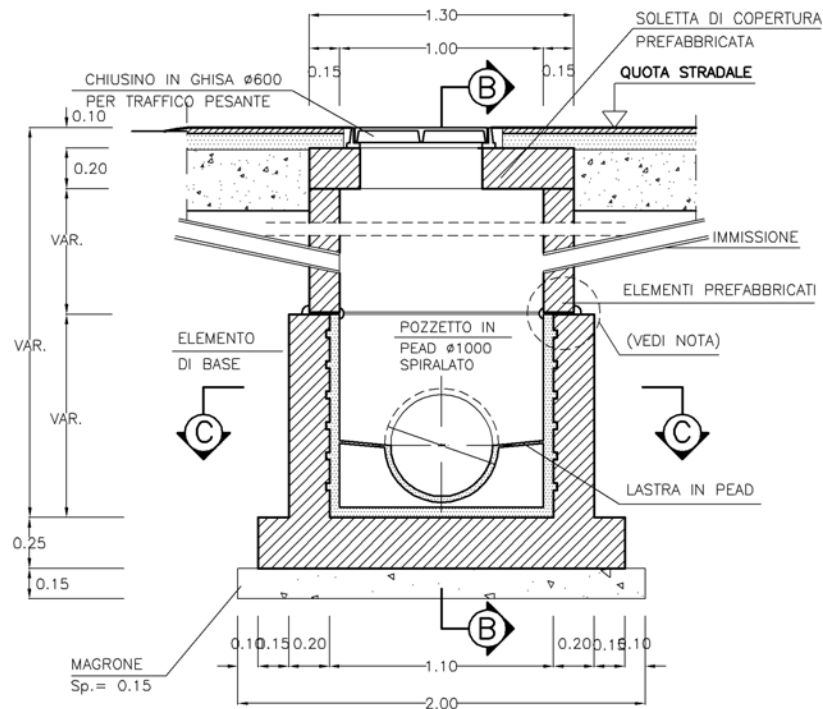
SEZIONE A-A 1:25
